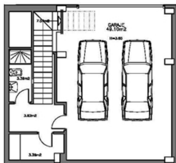
GARAJE DUPLEX E
